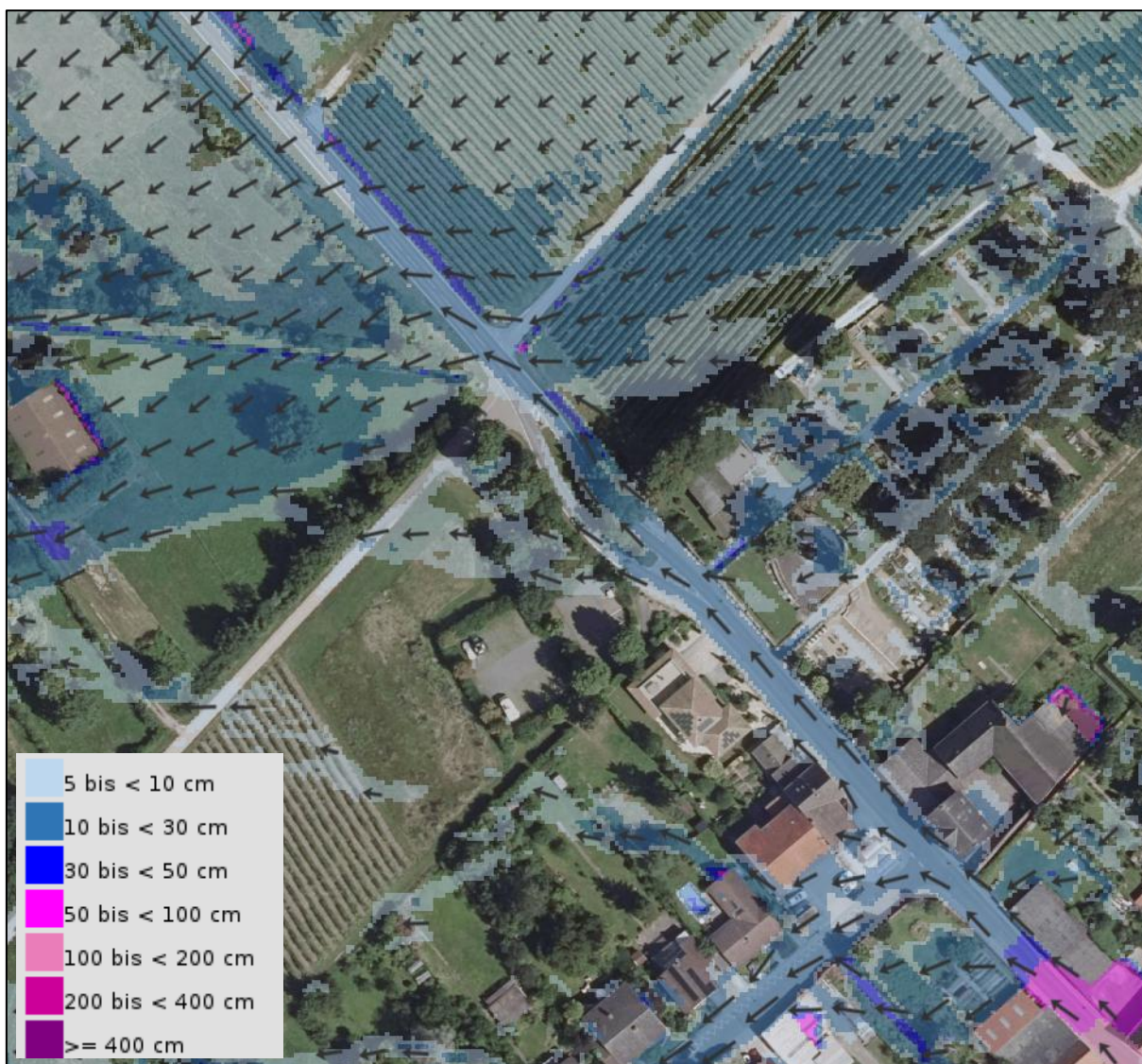
Abb. 10: Darstellung potenzieller Abflussrichtungen und Wassertiefen bei einem extremen Starkregenereignis (SRI 10, ca. 124–136 mm in vier Stunden) im Eingriffsbereich. Ausschnitt aus der Sturzflutgefahrenkarte: Herausgeber der Webseiten ist das Landesamt für Umwelt Rheinland-Pfalz (LfU) vertreten durch den Präsidenten des Landesamtes für Umwelt. Stand 09/25
