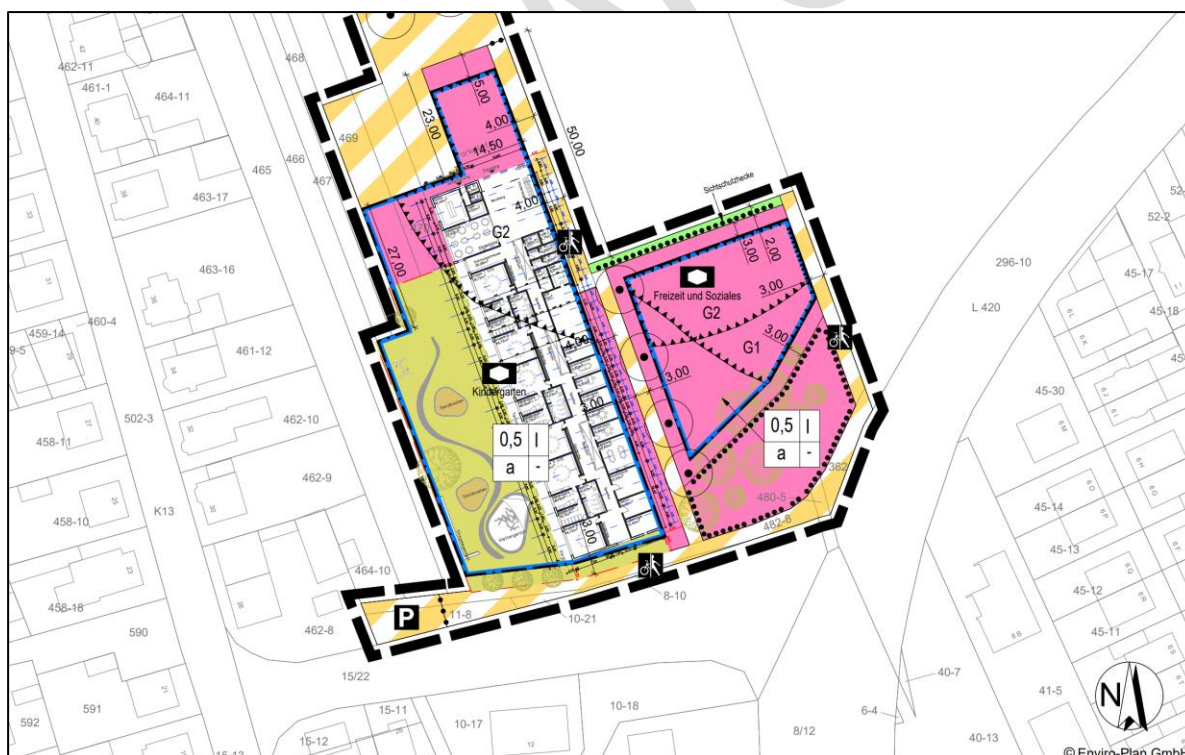
Abb. 7: Vorläufiger Entwurf des Baukörpers (erstellt durch Bau Eins Architekten PartGmbH, Kaiserslautern, 11.02.2025) in der Planzeichnung des Bebauungsplanentwurfs (erstellt durch Enviro-Plan GmbH, Odernheim am Glan, 11.06.2025); zusammengeführt durch Enviro-Plan 2025
